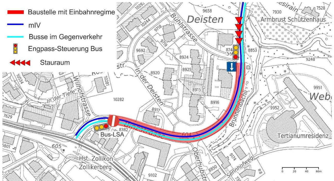
Verkehrsführung im Baustellenbereich (1. Etappe)
